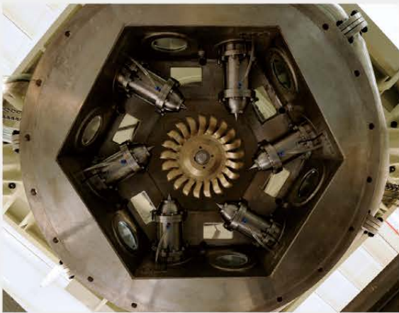
2020年12月1日，东方电机DF-300冲击式水力试验台顺利通过专家委员会验收。
