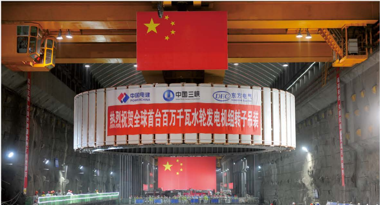
2020年08月18日，东方电机研制的全球首台白鹤滩1000MW水轮发电机组转子成功吊装。
